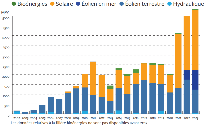
GRAPHIQUE 6 : ÉVOLUTION DE LA PUISSANCE RACCORDÉE PAR AN 358
