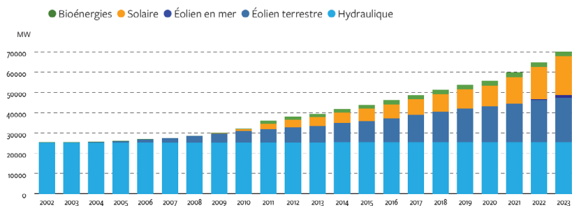
GRAPHIQUE 5 : EVOLUTION DE LA PUISSANCE INSTALLÉE 356
